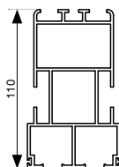
Profilo guida AG015
