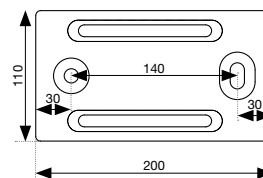
Staffa di premontaggio AG009
