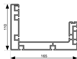
Profilo gronda AG002
