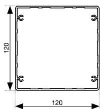
Profilo colonna AC430
