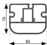
Frangitratta terminale AG005
