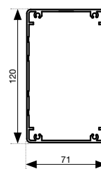
Profilo tettuccio AG019
