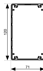
Profilo tettuccio AG019
